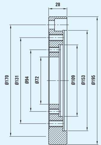
Промежуточный фланец Код 070700550
