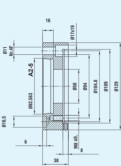
Фланец А2-5 Код 070700558
