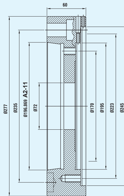
Фланец А2-11 Код 070700559
